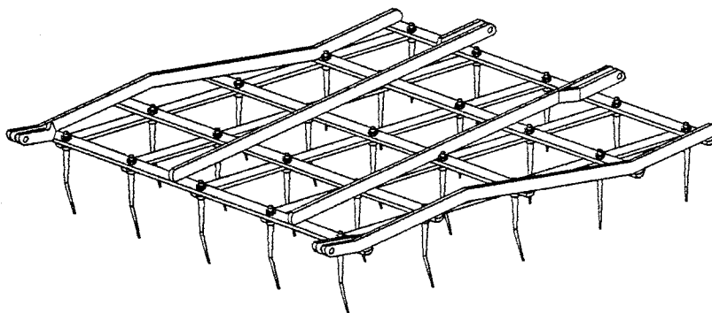
Eggenfeld Typ III m. Eggenzinken
