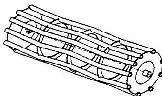
Rohrwalze \phi 330\text{mm} 9 Sprossen
