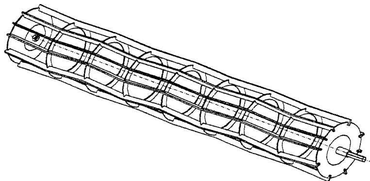
Sprossenwalze \phi 420\text{mm} 9 Sprossen, FL 8mm
