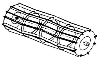
Sprossenwalze \phi 330\text{mm} 9 Sprossen, FL 8mm
