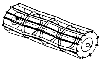
Sprossenwalze \phi 330\text{mm} 9 Sprossen, FL 6mm
